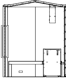
vista laterale
